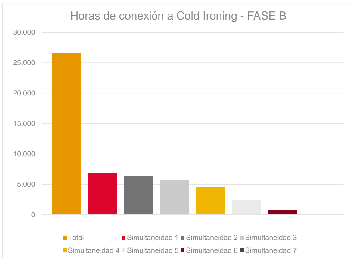
Figura 7. Distribución de horas de conexión a Cold Ironing en la fase B
