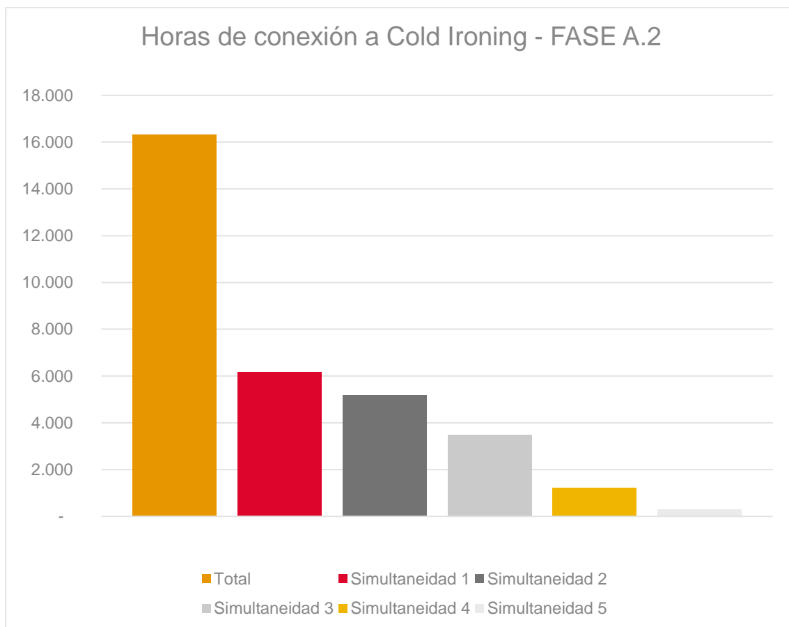
Figura 5. Distribución de horas de conexión a Cold Ironing en la fase A.2
